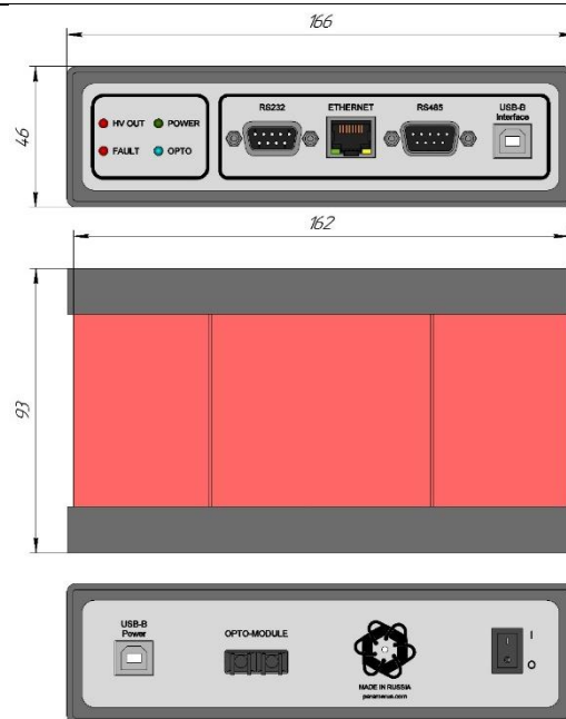
Рисунок 3. Габаритные размеры оптомодуля
