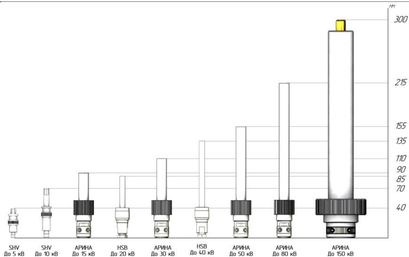
Рисунок 4. Номинальное напряжение и габаритные размеры высоковольтных разъемов.
