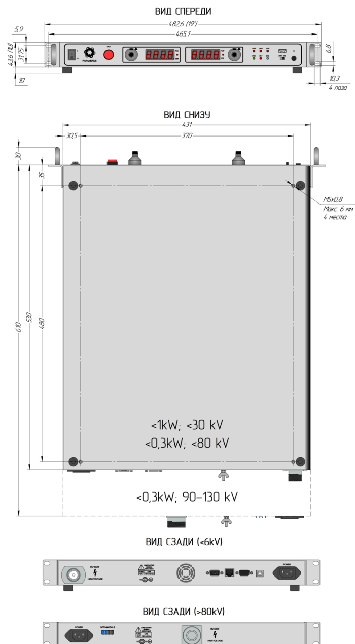
Рисунок 1. Габаритные размеры источников питания серии SHVLP в корпусе стандарта 1U и 2U
