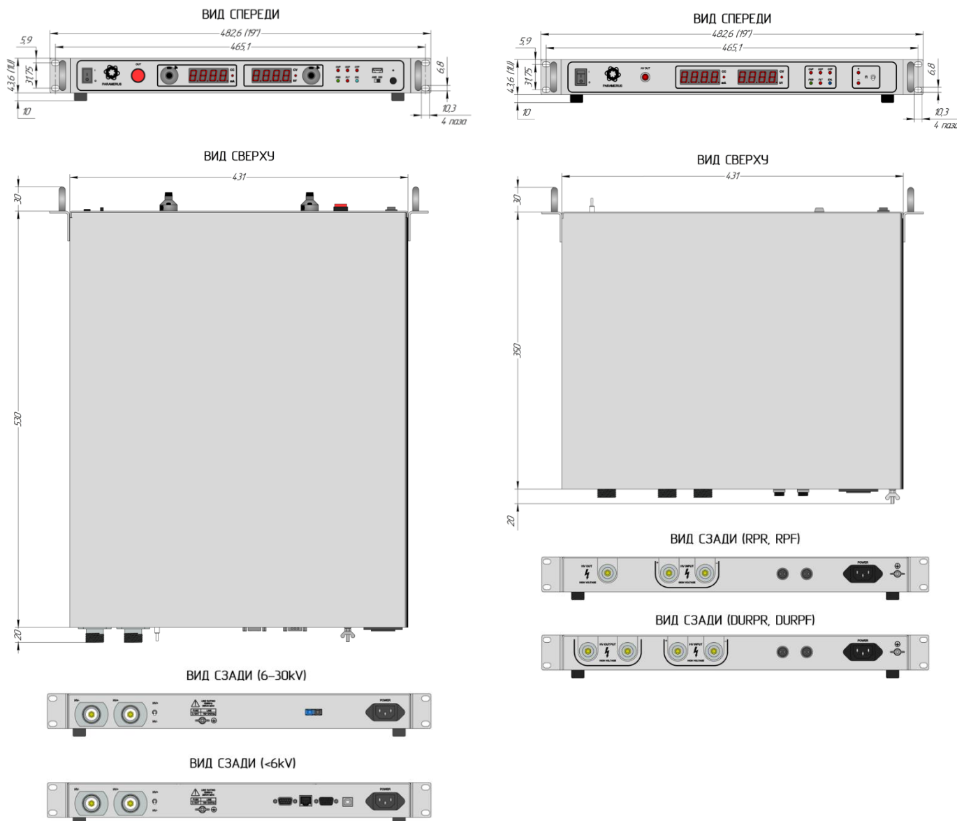
Рисунок 2. Габаритные размеры источников серии SHVLP-RP и релейного модуля HV-Relay
